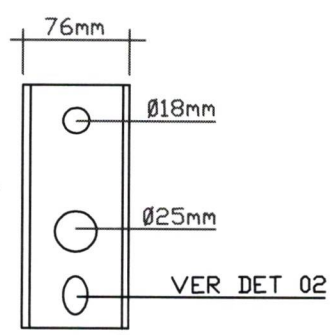
DET. 01
