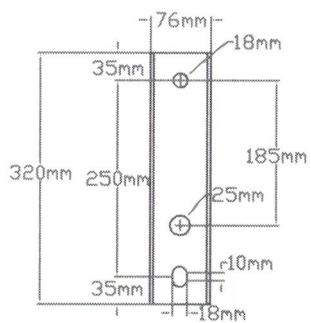
DETALHE DA BASE
