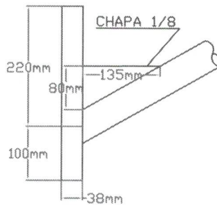
DETALHE DA BASE DE FIXAÇÃO PERFIL 1ª ALHA (4mm)
